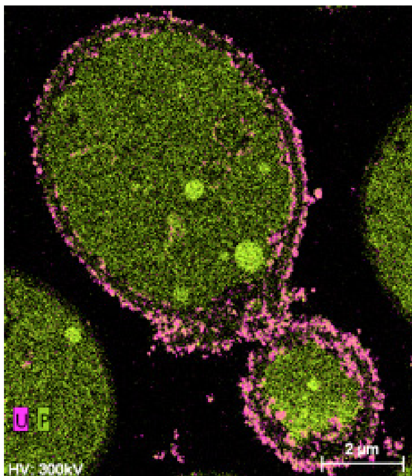
Figura 1. Ejemplo de biomineralización microbiana de fosfatos de uranio como estrategia de remediación de este metal pesado (Lopez-Fernandez et al. 2014).
